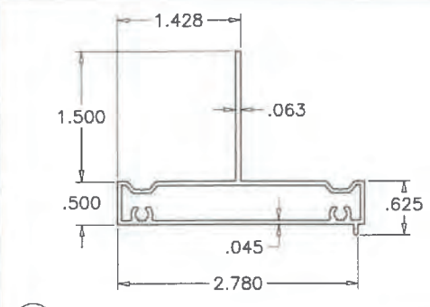
E15 FLUSH FRAME ADAPTER WITH FIN
