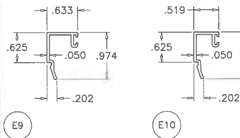
E9 E10 E10A GLAZING BEADS
