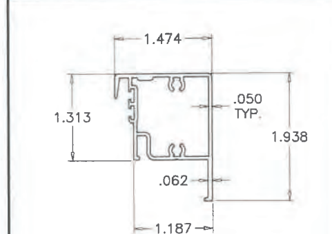
E5 VENT TOP RAIL
