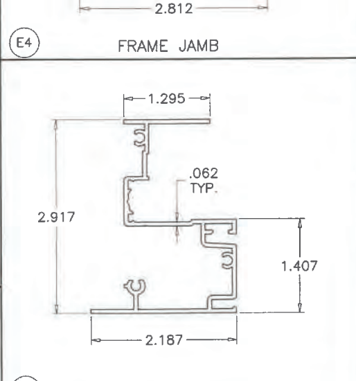
E4A ALT. FRAME JAMB
