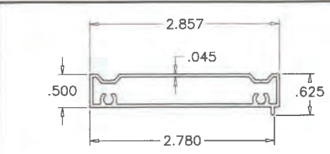
E12 FLUSH FRAME ADAPTER
