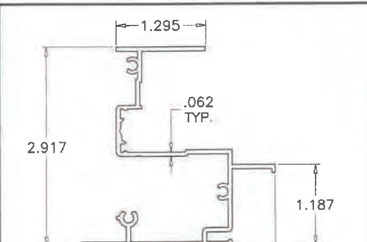
E4 FRAME JAMB
