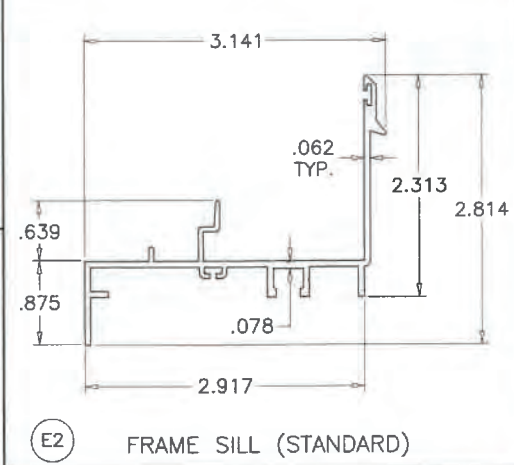
E2 FRAME SILL (STANDARD)
