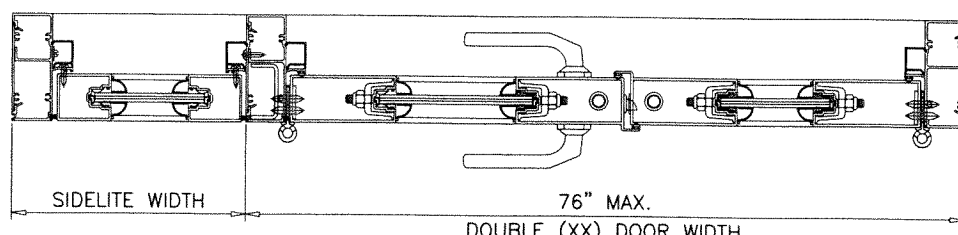
DOUBLE (XX) DOOR WIDTH
