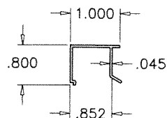
⑬ JAMB TRIM (OPTIONAL)
