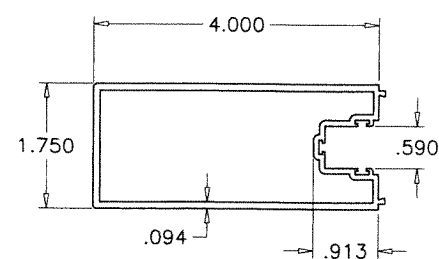
⑦ HINGE STILE
